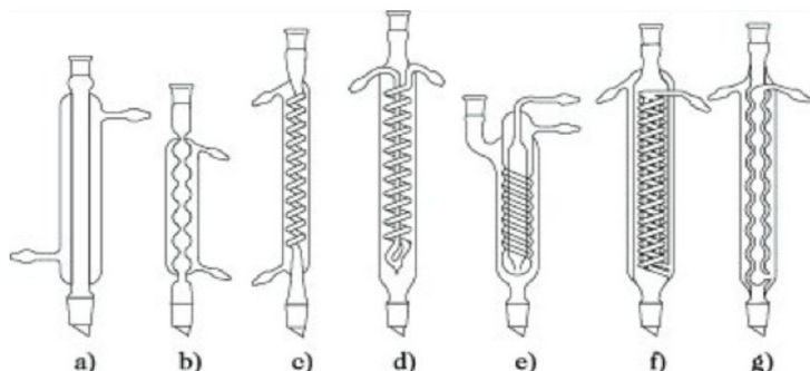
Kühler. Abb. 1: Im Labor verwendete Kühler: (a) Liebig-Kühler, (b) Kugelkühler, (c) Schlangenkühler, (d) Dimroth-Kühler, (e) Spiralkühler, (f) Doppelspiralkühler, (g) Wellrohrkühler.
